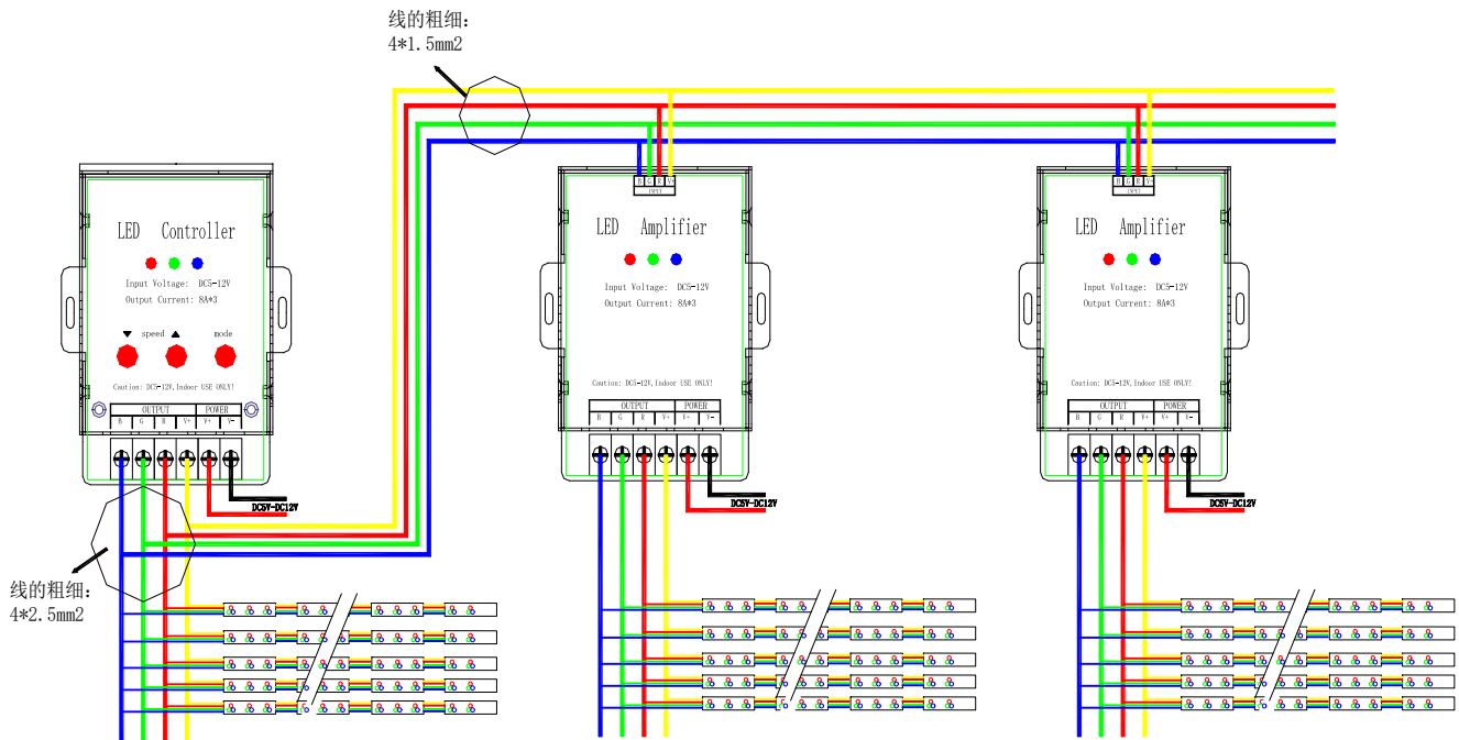
控制器与放大器接线示意图
